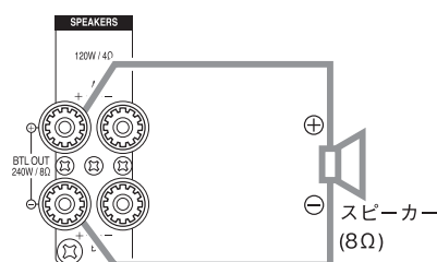
■図5 BTL設定時のスピーカー接続方法
