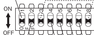
制御基板の 設定スイッチA
