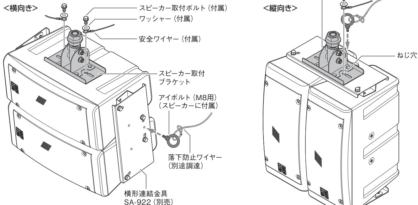
図 2 ※HMB-80HA2台をSA-922(別売)で連結した場合の図です。
