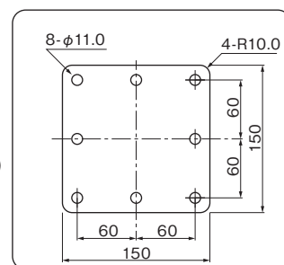
図 4 取付部寸法図
