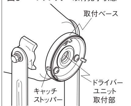
図3 レфлекター取付完了状態
