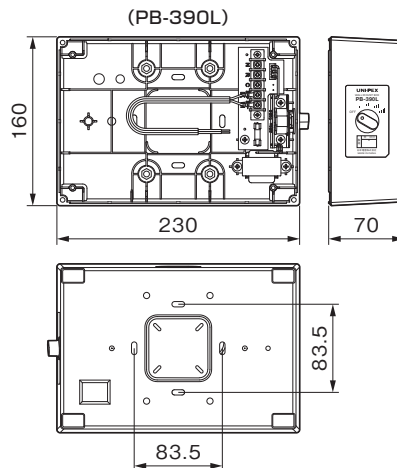
PL-392+PB-390L (組合せ例)
