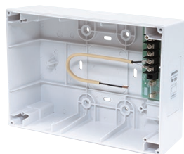
PB-390(ヒューズ付)
